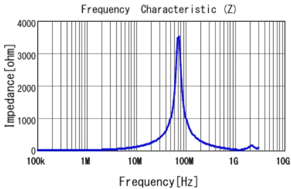
■ 1273AS-H-2R2N |Z|
