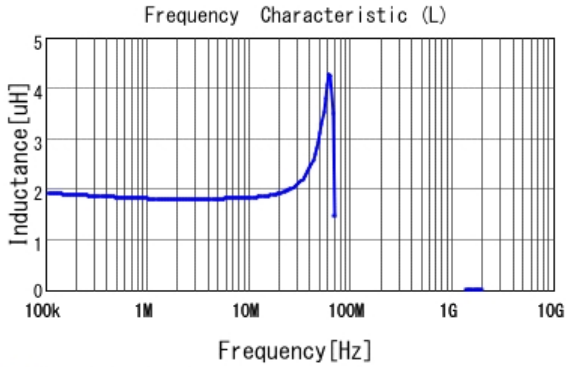
■ 1273AS-H-2R2N L
