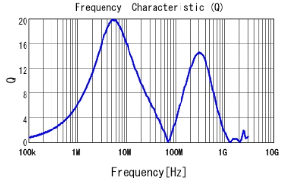
■ 1273AS-H-2R2N Q
